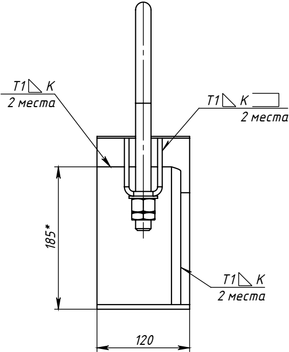
Поз.3 (Ложемент)
