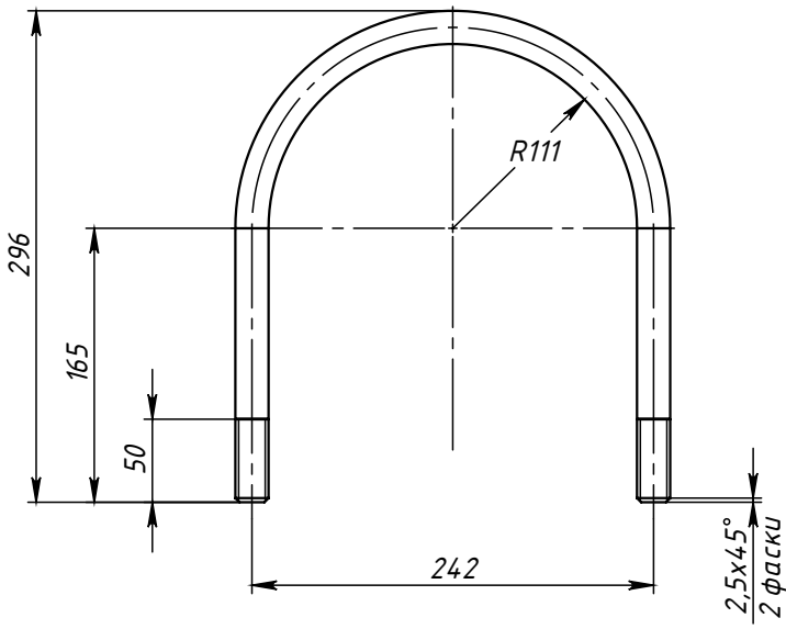
Поз.4 (Хомут)
